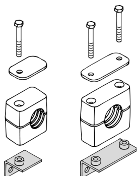
BASES DE SOLDA EM "L" TIPO WSP
