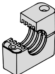
Desenho padrão – com desenho por dentro Folgas de tensão
