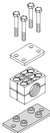
BASES DE SOLDA ALONGADAS PARA ABRAÇADEIRAS DUPLAS TIPO SPAS/DUEB
